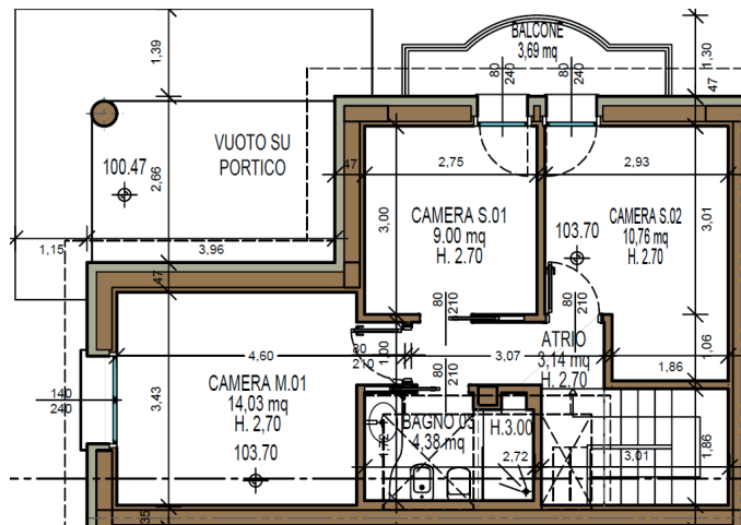
PIANO PRIMO QUOTATO
