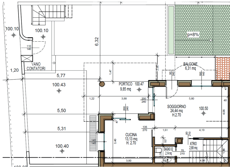
PIANO TERRA QUOTATO
