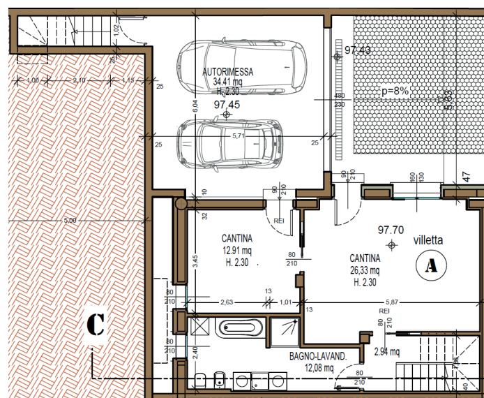
PIANO INTERRATO QUOTATO
